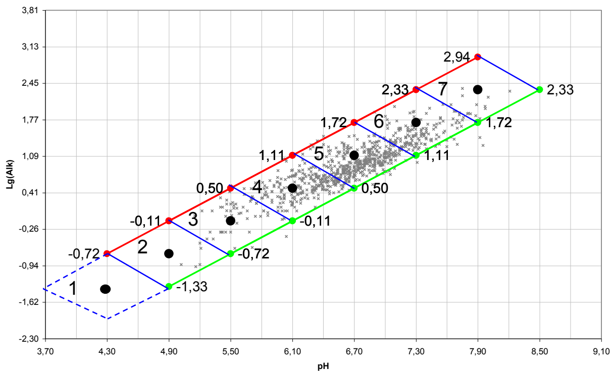
Рис. 2. Классификация водных объектов по рН и щелочности
